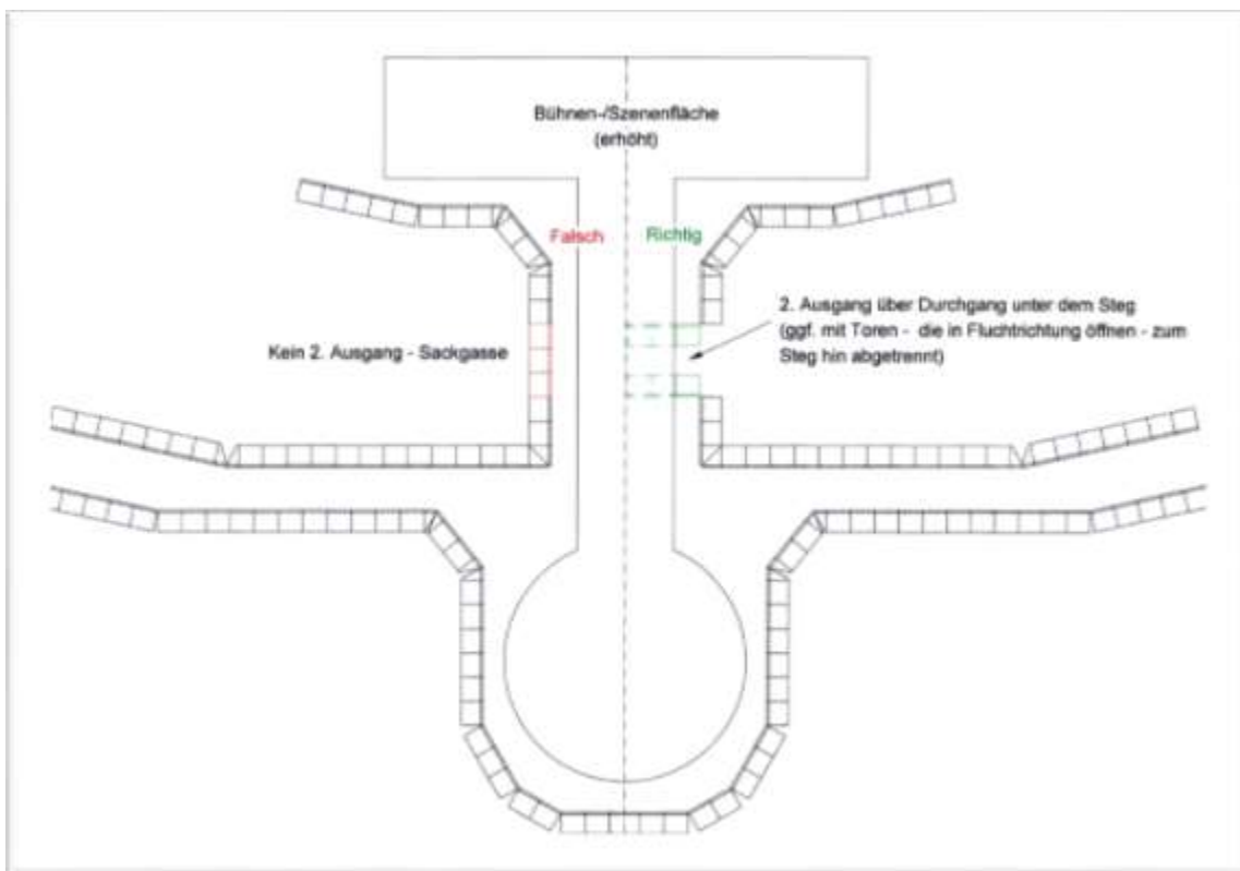
Abb. 26: Grundsatz der zwei Rettungswege (inkl. Vermeidung spitzer Winkel; entsprechende Durchgangshöhe wird für den unter der Bühne durchgehenden 2. Ausgang vorausgesetzt)
