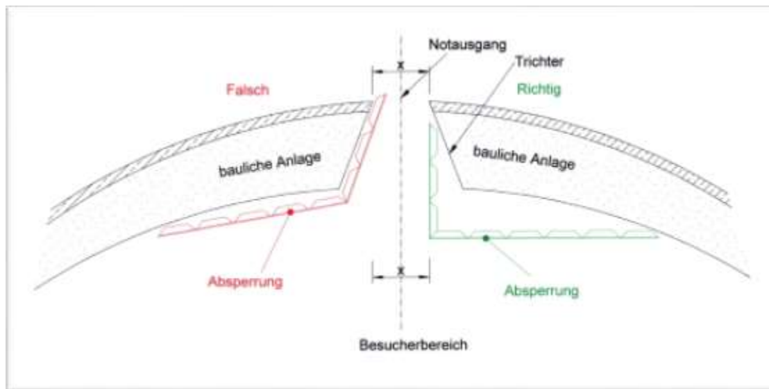
Abb.27: Vermeidung von Trichtern
