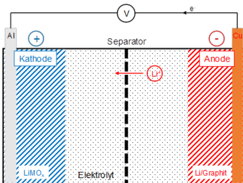
Abbildung 1: Schematische Darstellung des Aufbaus einer sekundären Lithium-Ionen-Batterie beim Entladevorgang (Quelle: Referat 10 vfdb)
