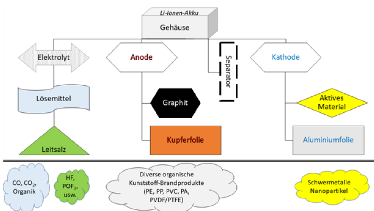
Abbildung 3: Zusammensetzung und Gefahrstoffe beim Brand von Lithium-Batterien (Quelle: Referat 10 vfdb)
